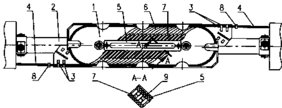
Рис. 5. Заведение модулей, раскладка ОВ и установка гильз КДЗС в кассете. 1) Кассета. 2) Лоток. 3) Стяжка нейлоновая. 4) Пучки модульных трубок. 5) Планка прижимная. 6) Оптическое волокно. 7) Гильза КДЗС. 8) Маркеры. 9) Уплотнение.
