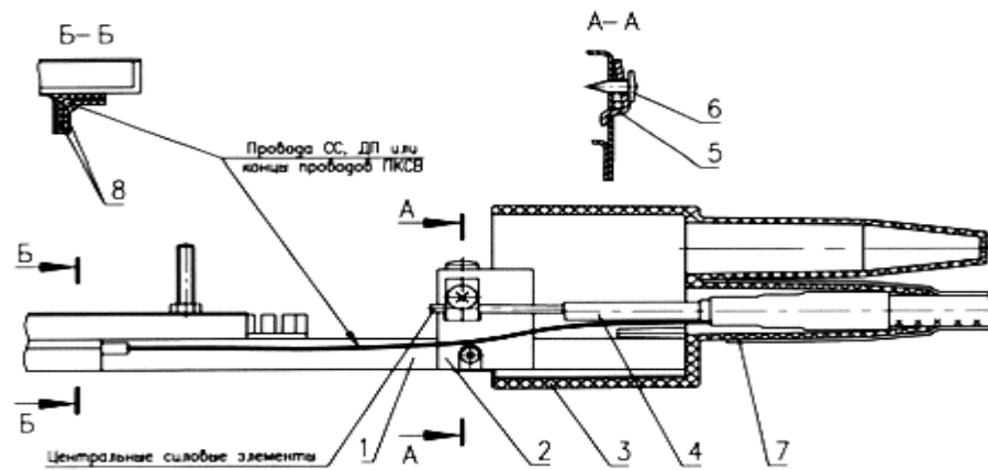
Рис. 4. Закрепление концов кабеля, центрального силового элемента, проводов СС и ДП или проводов ПКСВ 1) Лоток. 2) Кронштейн лотка. 3) Оголовник. 4) Кабель. 5) Пластина ЦСЭ. 6) Винт. 7) Трубка ТУТ 35/12. 8) Пластина МГ.
