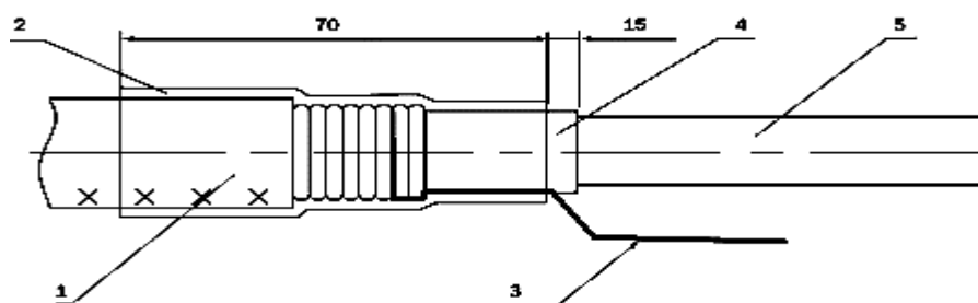
Рис. 3. Продольная герметизация кабеля.
