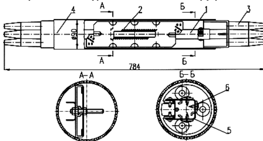
Рис. 1. Муфта оптическая городская укороченная (МОГ-С) 1) Лоток. 2) Кассета типа К. 3) Оголовник. 4) Труба. 5) Кронштейн лотка. б) Узел закрепления ЦСЭ.
