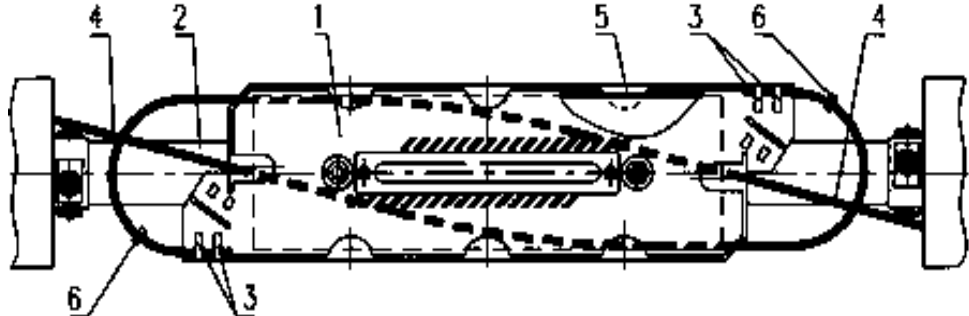
Рис. 6. Заведение модулей на дополнительную кассету. 1) Кассета. 2) Лоток. 3) Стяжка нейлоновая. 4) Пучки модульных трубок. 5) Подкассетник. 6) Маркеры.
