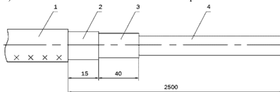
Рис. 2. Разделка оптического кабеля с любым бронепокровом 1) Кабель. 2) Бронепокров. 3) Промежуточная оболочка. 4) Модули.
