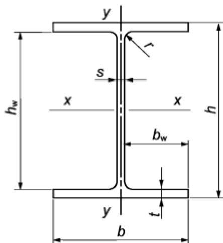
Рисунок 1. Двутавр.
