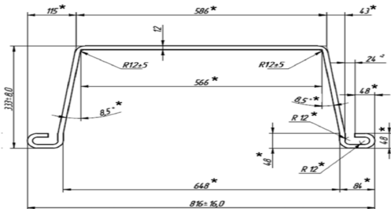
Рисунок 1 - Поперечное сечение GRANI тип 1
