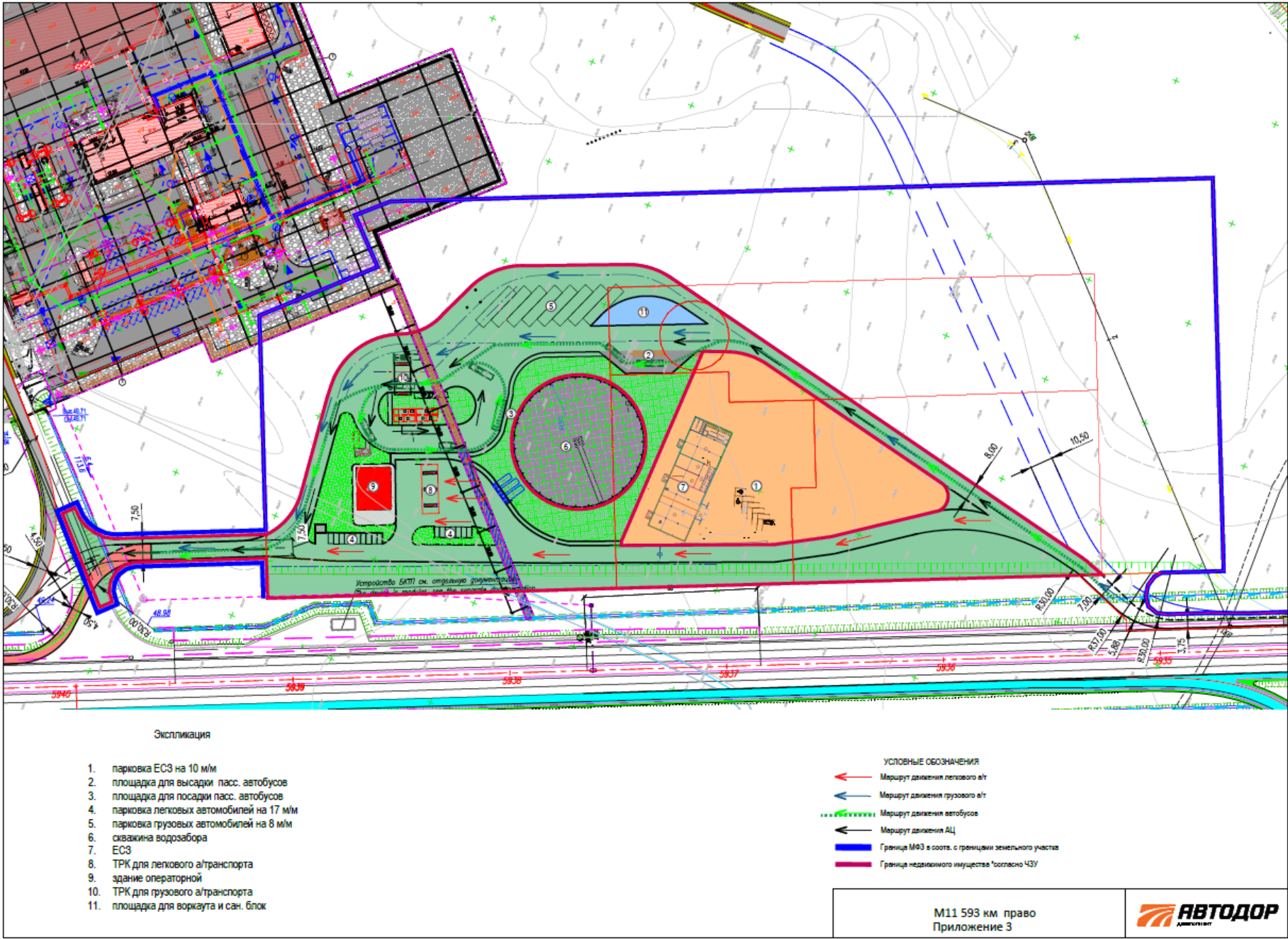
Схема застройки многофункциональной зоны дорожного сервиса
